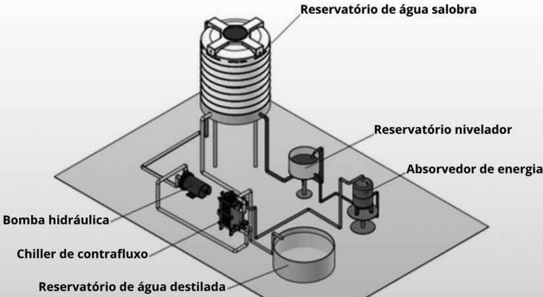
Inovação baseia-se na mudança de fase da água, explorando o processo de evaporação induzido pela energia solar
